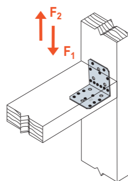
SCHEMAT OBCIĄŻENIA połączenie belka-słup ramię skierowane w górę
