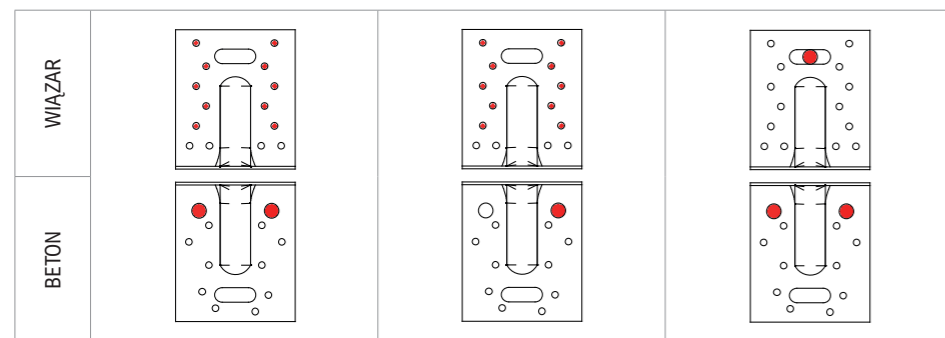
SCHEMAT 1 POŁĄCZENIE WIĄZAR - BETON SCHEMAT 2 POŁĄCZENIE WIĄZAR - BETON SCHEMAT 3 POŁĄCZENIE WIĄZAR - BETON
