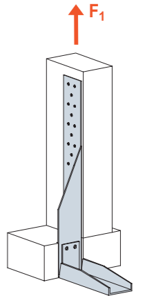
SCHEMAT OBCIĄŻENIA połączenie słup- beton
