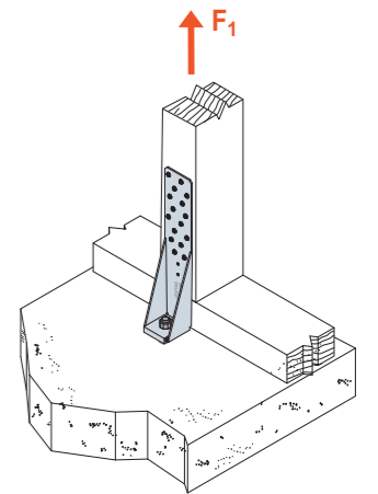
SCHEMAT OBCIĄŻENIA połączenie słup- beton
