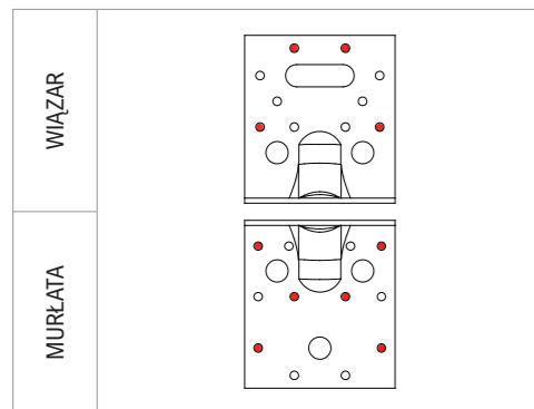
SCHEMAT GWOŹDZIOWANIA CZĘŚCIOWEGO POŁĄCZENIE WIĄZAR-MURŁATA
