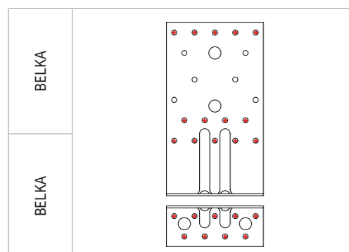
SCHEMAT GWOŹDZIOWANIA CZĘŚCIOWEGO POŁĄCZENIE BELKA-BELKA
