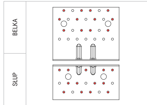
SCHEMAT GWOŹDZIOWANIA CZĘŚCIOWEGO POŁĄCZENIE BELKA-SŁUP
