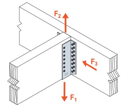
SCHEMAT OBCIĄŻENIA połączenie belka-belka
