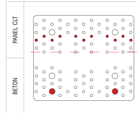
SCHEMAT GWOŹDZIOWANIA NPB255 POŁĄCZENIE PANEL CLT - BETON
