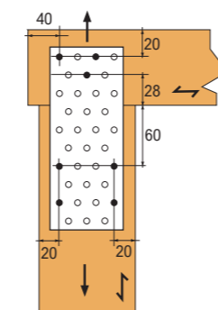
Minimalne odległości od końca i boku elementu
