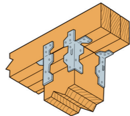
Połączenie belka-słup
