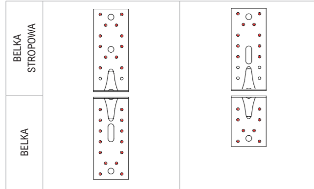
SCHEMAT POŁĄCZENIA BELKA-BELKA STROPOWA
