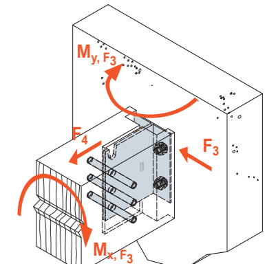
SCHEMAT OBCIĄŻENIA połączenie belka- beton
