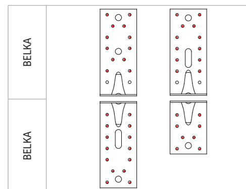
SCHEMAT GWOŹDZIOWANIA PEŁNEGO POŁĄCZENIE BELKA-BELKA
