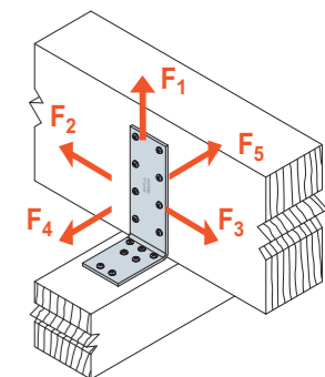
SCHEMAT OBCIĄŻENIA połączenie belka-belka dwa złącza na połączenie
