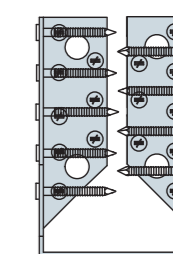
Gwoździowanie pełne
