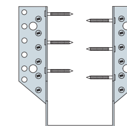
Gwoździowanie częściowe
