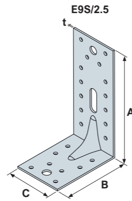
E9S/2,5
