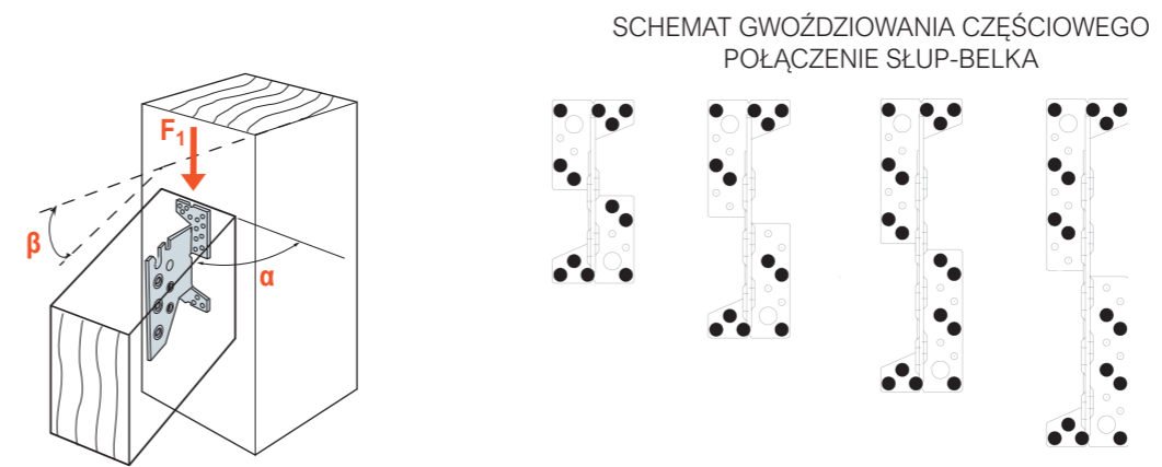
SCHEMAT OBCIĄŻENIA połączenie belka-słup
