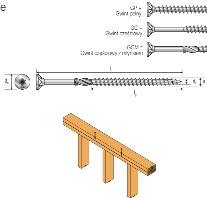
Przykład połączenia oczepu za pomocą wkrętów TTUFS
