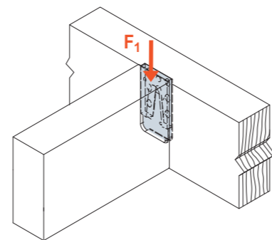
SCHEMAT OBCIĄŻENIA połączenie belka- belka
