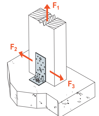
SCHEMAT OBCIĄŻENIA połączenie słup-beton dwa złącza na połączenie
