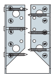
Gwoździowanie częściowe
