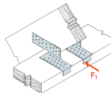
SCHEMAT OBCIĄŻENIA połączenie belka - belka
