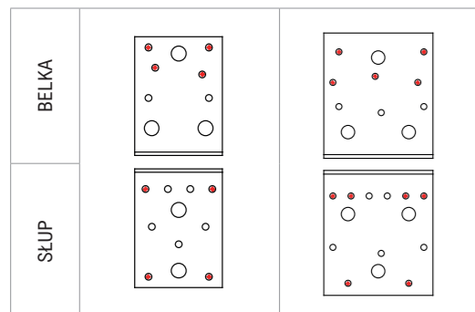
SCHEMAT GWOŹDZIOWANIA CZĘŚCIOWEGO POŁĄCZENIE BELKA - SŁUP
