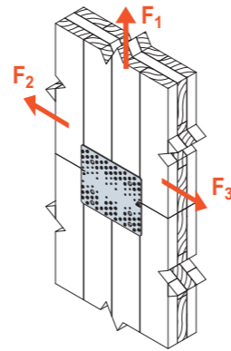
SCHEMAT OBCIĄŻENIA połączenie CLT - CLT
