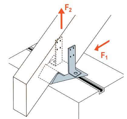
SCHEMAT OBCIĄŻENIA połączenie krokiew - wieniec
