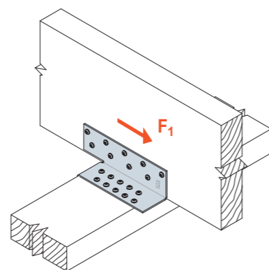
SCHEMAT OBCIĄŻENIA połączenie belka - belka
