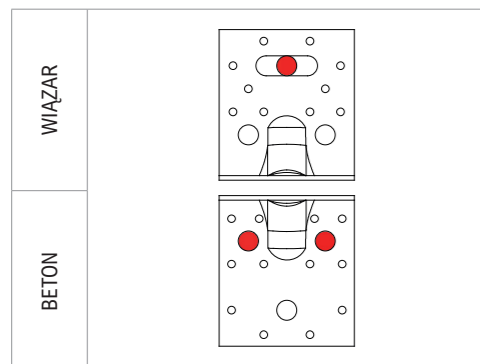
SCHEMAT POŁĄCZENIA WIĄZAR-BETON
