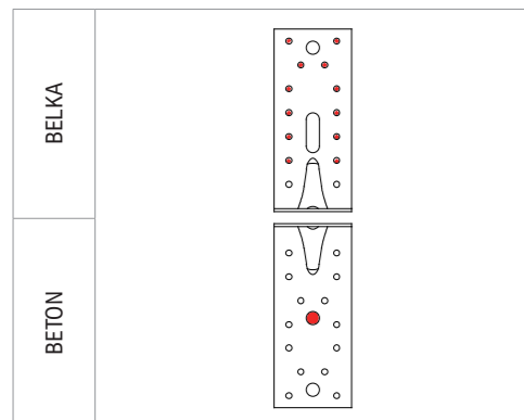
SCHEMAT POŁĄCZENIA BELKA-BETON
