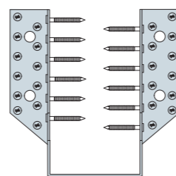
Gwoździowanie pełne
