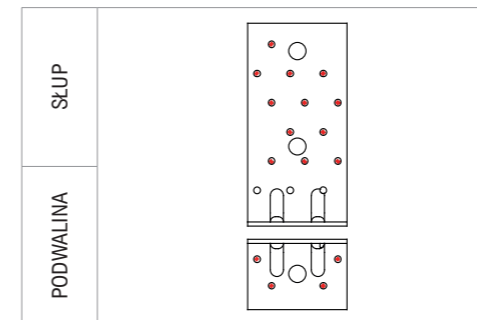
SCHEMAT GWOŹDZIOWANIA PEŁNEGO POŁĄCZENIE SŁUP-PODWALINA
