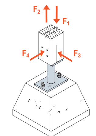
SCHEMAT OBCIĄŻENIA połączenie słup- beton
