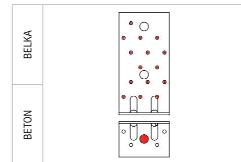
SCHEMAT GWOŹDZIOWANIA PEŁNEGO POŁĄCZENIE BELKA-BETON
