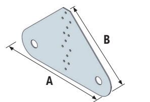
Błacha węzłowa BNK25
