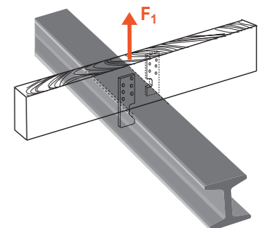
SCHEMAT OBCIĄŻENIA połączenie belka - belka stalowa
