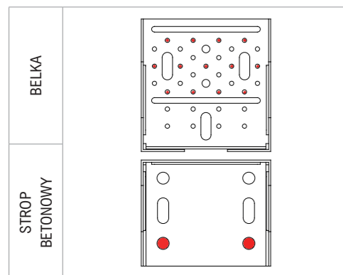
SCHEMAT GWOŹDZIOWANIA CZĘŚCIOWEGO POŁĄCZENIE BELKA-STROP BETONOWY
