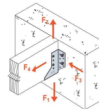
SCHEMAT OBCIĄŻENIA połączenie belka-ściana betonowa
