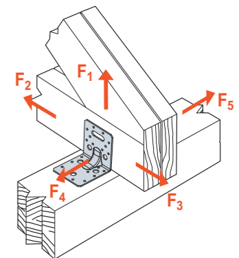
SCHEMAT OBCIĄŻENIA połączenie więźar-murłata dwa złącza na połączenie
