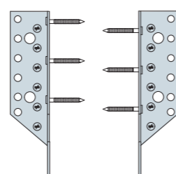
Gwoździowanie częściowe
