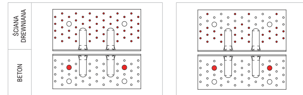
SCHEMAT GWOŹDZIOWANIA PEŁNEGO POŁĄCZENIE ŚCIANA CLT-BETON
