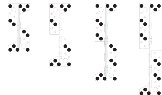
SCHEMAT GWOŹDZIOWANIA CZĘŚCIOWEGO POŁĄCZENIE SŁUP-BELKA
