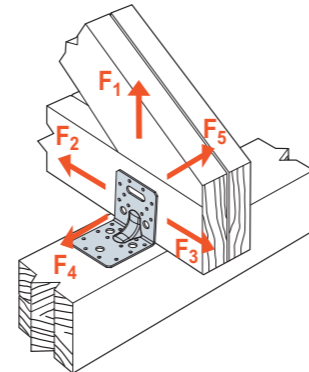
SCHEMAT OBCIĄŻENIA połączenie więźar-murłata dwa złącza na połączenie
