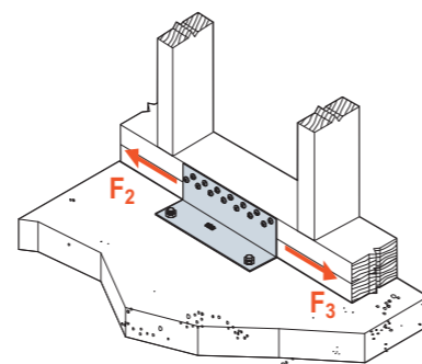
SCHEMAT OBCIĄŻENIA połączenie ściana szkieletowa-beton jedno złącze na połączenie
