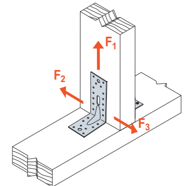
SCHEMAT OBCIĄŻENIA połączenie słup-podwalina dwa złącza na połączenie
