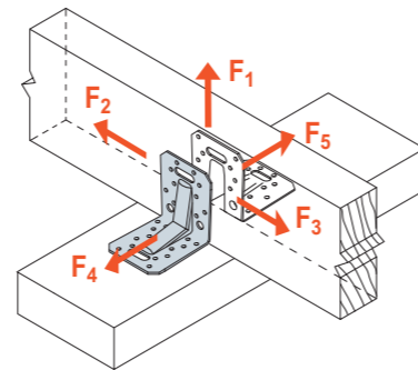
SCHEMAT OBCIĄŻENIA połączenie więźar-murłata dwa złącza na połączenie
