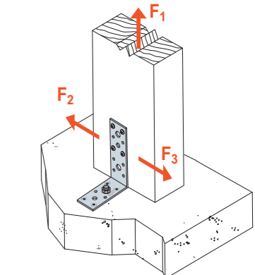
SCHEMAT OBCIĄŻENIA połączenie słup-beton dwa złącza na połączenie
