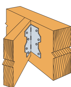
SCHEMAT OBCIĄŻENIA połączenie belka - belka
