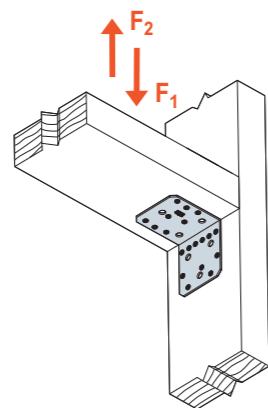
SCHEMAT OBCIĄŻENIA połączenie belka-słup ramię skierowane w dół
