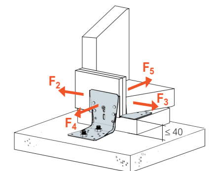
SCHEMAT OBCIĄŻENIA połączenie belka- beton
