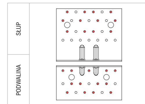
SCHEMAT GWOŹDZIOWANIA CZĘŚCIOWEGO POŁĄCZENIE SŁUP-PODVALINA
