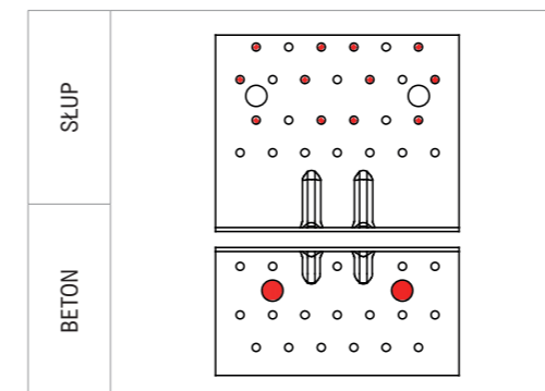
SCHEMAT GWOŹDZIOWANIA CZĘŚCIOWEGO POŁĄCZENIE SŁUP-BETON
