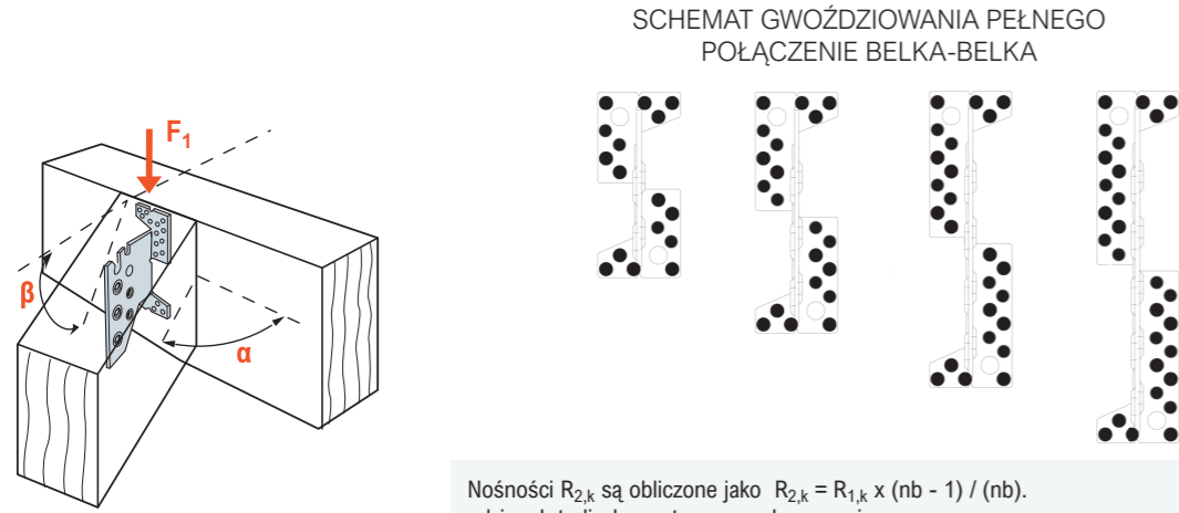
SCHEMAT OBCIĄŻENIA połączenie belka- belka
