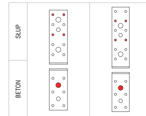
SCHEMAT GWOŹDZIOWANIA CZĘŚCIOWEGO POŁĄCZENIE SŁUP-BETON
