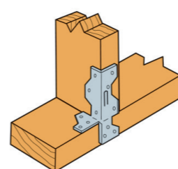
Połączenie słup-podwalina
