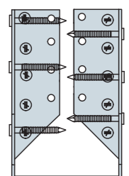
Gwoździowanie częściowe
