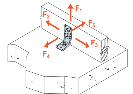
SCHEMAT OBCIĄŻENIA połączenie belka- beton
