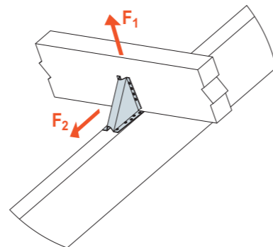
SCHEMAT OBCIĄŻENIA połączenie belka-belka jedno złącze na połączenie
