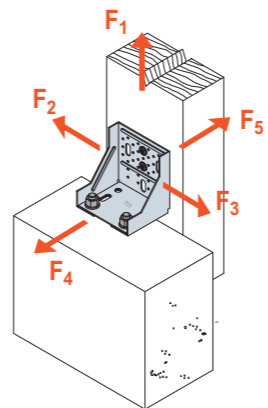
SCHEMAT OBCIĄŻENIA połączenie belka-strop betonowy
