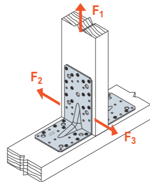
SCHEMAT OBCIĄŻENIA połączenie słup-podwalina dwa złącza na połączenie
