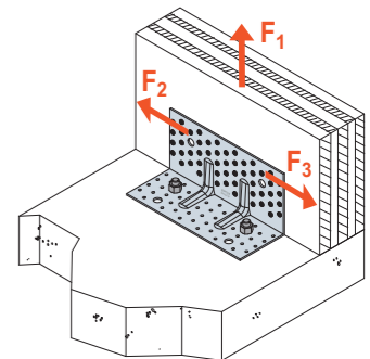
SCHEMAT OBCIĄŻENIA połączenie ściana CLT-beton jedno złącze na połączenie
