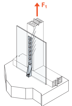
SCHEMAT OBCIĄŻENIA połączenie słup- beton
