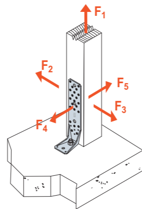
SCHEMAT OBCIĄŻENIA połączenie słup- beton
