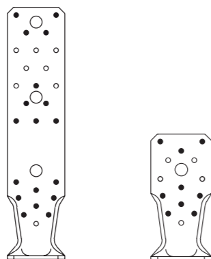
SCHEMAT GWOŹDZIOWANIA CZĘŚCIOWEGO POŁĄCZENIE BELKA-BETON
