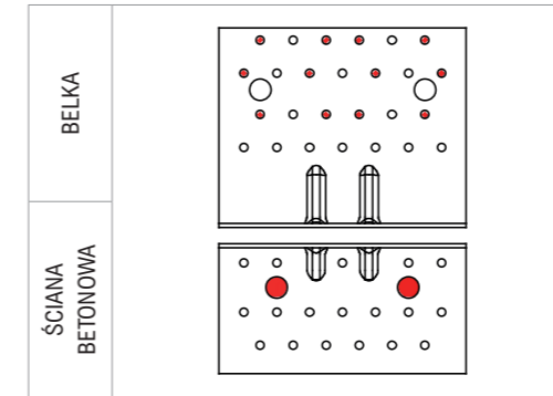
SCHEMAT GWOŹDZIOWANIA CZĘŚCIOWEGO POŁĄCZENIE BELKA-ŚCIANA BETONOWA
