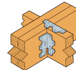
Połączenie belka-belka
