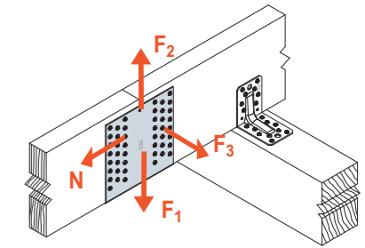
SCHEMAT OBCIĄŻENIA połączenie belka - belka
