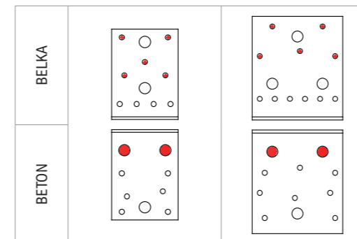
SCHEMAT GWOŹDZIOWANIA CZĘŚCIOWEGO POŁĄCZENIE BELKA - BETON
