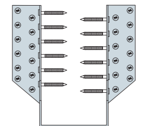
Gwoździowanie pełne
