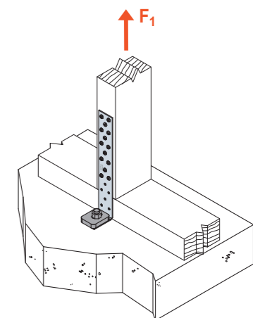
SCHEMAT OBCIĄŻENIA połączenie słup- beton
