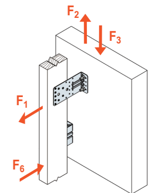
SCHEMAT OBCIĄŻENIA połączenie belka-beton fasada
