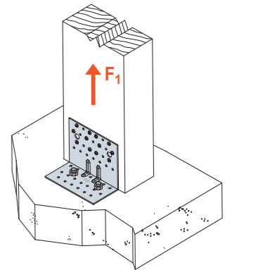
SCHEMAT OBCIĄŻENIA połączenie słup-beton dwa złącza na połączenie
