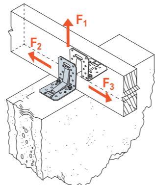
SCHEMAT OBCIĄŻENIA połączenie więźar- beton dwa złącza na połączenie
