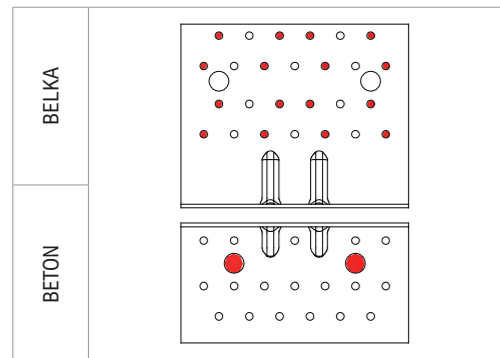
SCHEMAT GWOŹDZIOWANIA CZĘŚCIOWEGO POŁĄCZENIE BELKA-BETON
