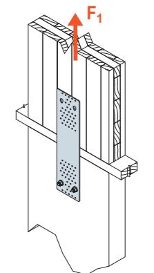
SCHEMAT OBCIĄŻENIA połączenie panel CLT - beton
