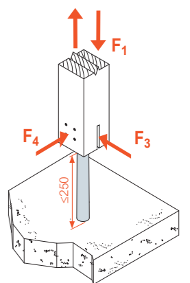
SCHEMAT OBCIĄŻENIA połączenie słup- beton
