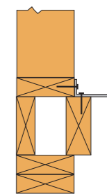
SCHEMAT OBCIĄŻENIA połączenie ściana szkieletowa-strop jedno złącze na połączenie
