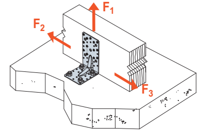
SCHEMAT OBCIĄŻENIA połączenie belka-beton dwa złącza na połączenie
