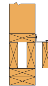
SCHEMAT POŁĄCZENIA -1 POŁĄCZENIE ŚCIANA SZKIELETOWA-STROP
