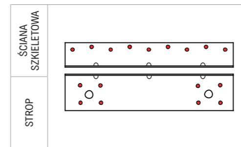
SCHEMAT GWOŹDZIOWANIA PEŁNEGO POŁĄCZENIE ŚCIANA SZKIELETOWA-STROP
