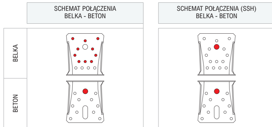
Połączenie drewnianej belki do betonu za pomocą kątownika ABR100.
