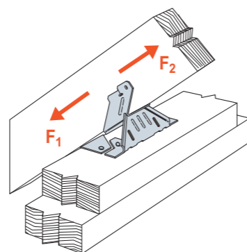
SCHEMAT OBCIĄŻENIA połączenie krokiew-murłata
