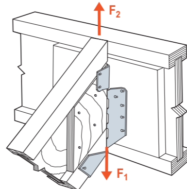
SCHEMAT OBCIĄŻENIA połączenie I-beam - I-beam
