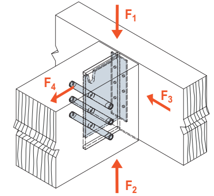
SCHEMAT OBCIĄŻENIA połączenie belka- belka
