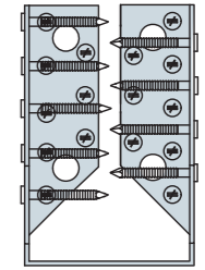
Gwoździowanie pełne
