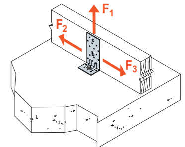
SCHEMAT OBCIĄŻENIA połączenie belka-beton dwa złącza na połączenie
