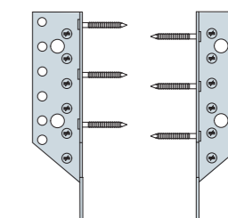
Gwoździowanie częściowe
