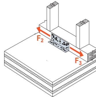
SCHEMAT OBCIĄŻENIA połączenie ściana szkieletowa-strop jedno złącze na połączenie
