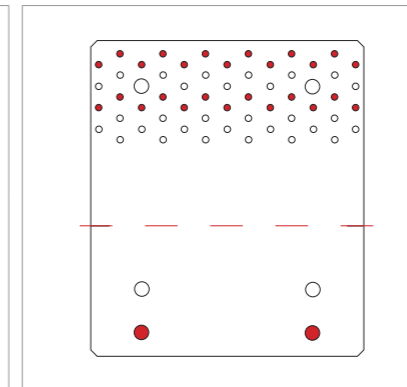
SCHEMAT GWOŹDZIOWANIA NPB255SO POŁĄCZENIE PANEL CLT - BETON
