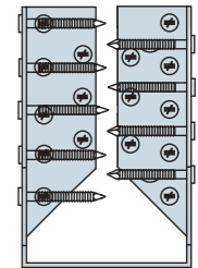
Gwoździowanie pełne
