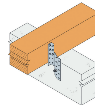
Połączenie belka-beton
