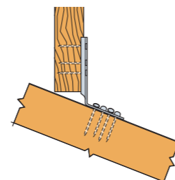
SCHEMAT OBCIĄŻENIA połączenie belka - wiązar
