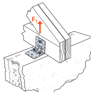
SCHEMAT OBCIĄŻENIA połączenie więźar-beton dwa złącza na połączenie
