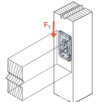
SCHEMAT OBCIĄŻENIA połączenie belka-słup
