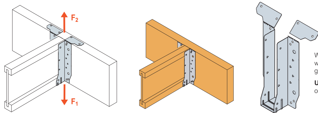
SCHEMAT OBCIĄŻENIA połączenie I-beam - belka
