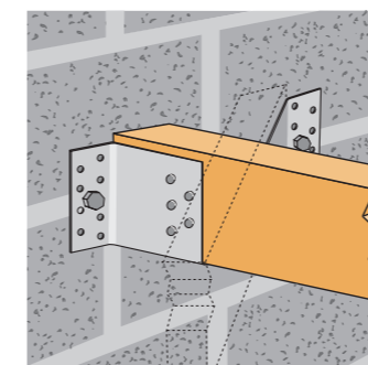
ET260
