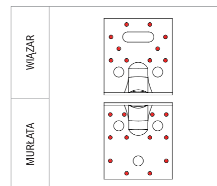
SCHEMAT GWOŹDZIOWANIA PEŁNEGO POŁĄCZENIE WIĄZAR-MURŁATA
