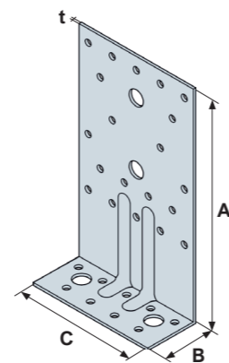
ABR220
