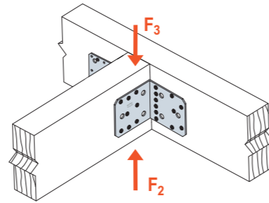
SCHEMAT OBCIĄŻENIA połączenie belka-belka stropowa dwa złącza na połączenie
