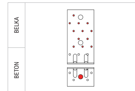
SCHEMAT GWOŹDZIOWANIA PEŁNEGO POŁĄCZENIE SŁUP-BETON
