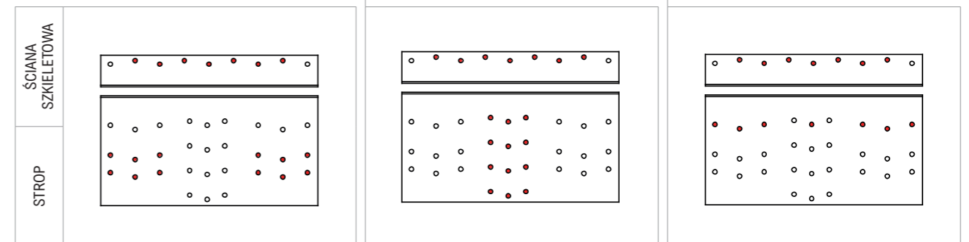
SCHEMAT POŁĄCZENIA -1 POŁĄCZENIE ŚCIANA SZKIELETOWA-STROP
