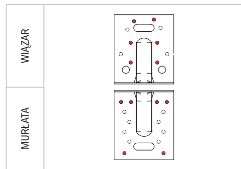
SCHEMAT GWOŹDZIOWANIA CZĘŚCIOWEGO POŁĄCZENIE WIĄZAR-MURŁATA
