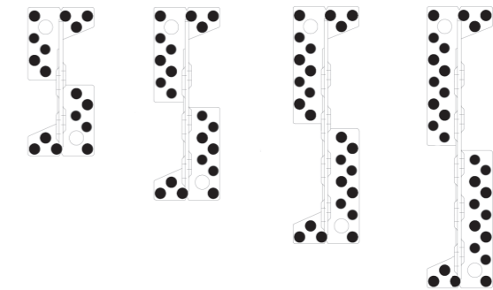
SCHEMAT GWOŹDZIOWANIA PEŁNEGO POŁĄCZENIE BELKA-BELKA
