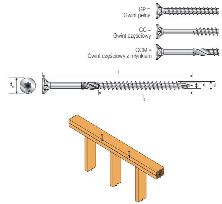
Przykłady połączenia oczepu za pomocą wkrętów TTZNFS
