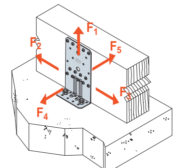
SCHEMAT OBCIĄŻENIA połączenie belka-beton dwa złącza na połączenie
