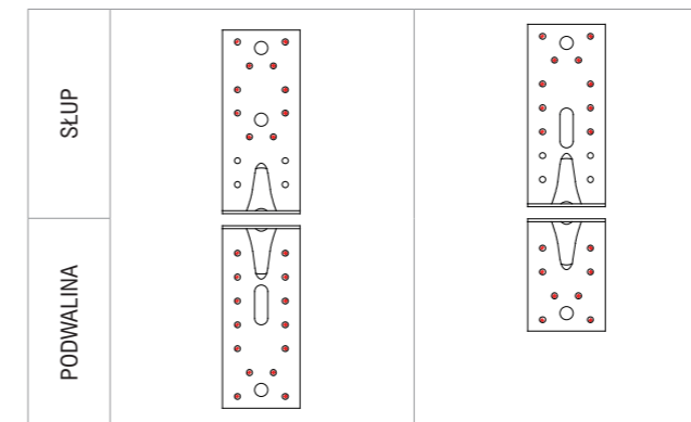
SCHEMAT GWOŹDZIOWANIA CZĘŚCIOWEGO POŁĄCZENIE SŁUP-PODWALINA
