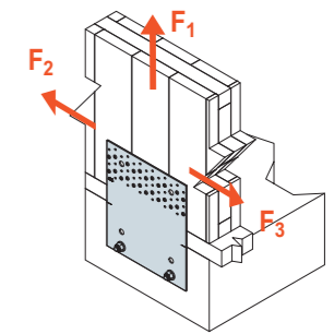
SCHEMAT OBCIĄŻENIA połączenie panel CLT - beton
