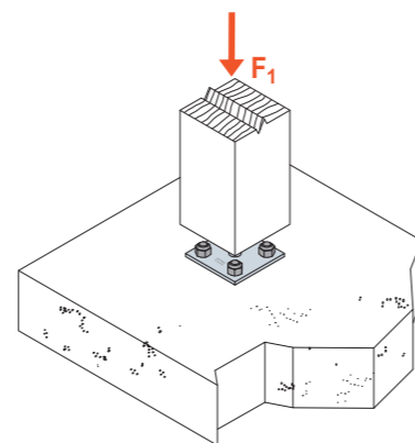
SCHEMAT OBCIĄŻENIA połączenie słu-p- beton
