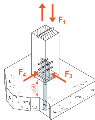
SCHEMAT OBCIĄŻENIA połączenie słup- beton
