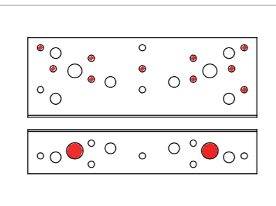
SCHEMAT POŁĄCZENIA -2 POŁĄCZENIE ŚCIANA SZKIELETOWA-BETON
