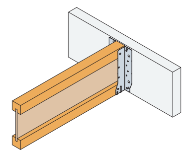
Połączenie doczołowe do betonu
