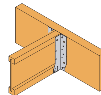
Połączenie doczołowe
