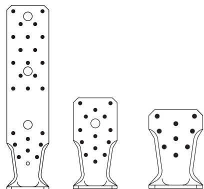
SCHEMAT GWOŹDZIOWANIA PEŁNEGO POŁĄCZENIE BELKA-BELKA
