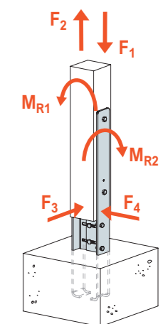
SCHEMAT OBCIĄŻENIA połączenie słup- beton
