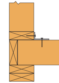
SCHEMAT POŁĄCZENIA -2 POŁĄCZENIE ŚCIANA SZKIELETOWA-STROP
