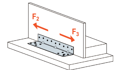
SCHEMAT OBCIĄŻENIA połączenie ściana szkieletowa-strop jedno złącze na połączenie
