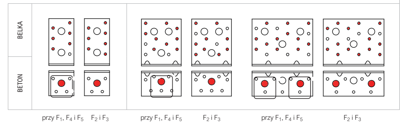
SCHEMAT POŁĄCZENIA BELKA - BETON
