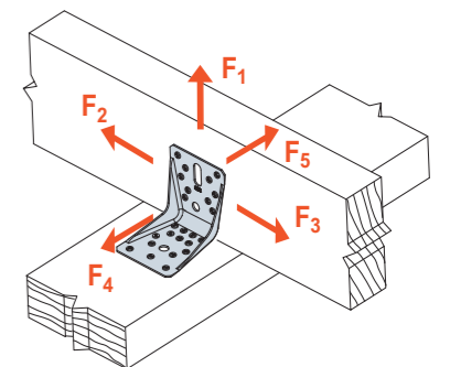
SCHEMAT OBCIĄŻENIA połączenie belka- belka dwa złącza na połączenie
