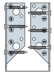
Gwoździowanie częściowe
