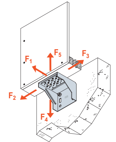
SCHEMAT OBCIĄŻENIA połączenie belka-ściana betonowa
