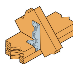
Połączenie krokiew-oczep
