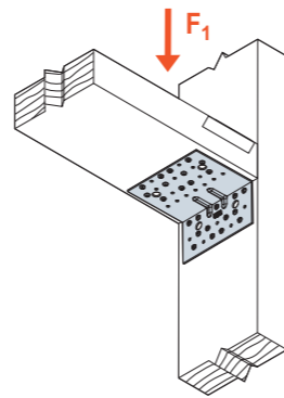
SCHEMAT OBCIĄŻENIA połączenie belka-słup jedno złącze na połączenie
