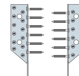
Gwoździowanie pełne
