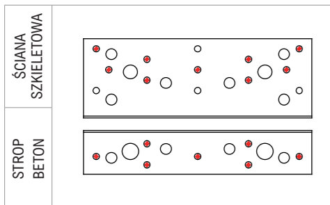
SCHEMAT POŁĄCZENIA -1 POŁĄCZENIE ŚCIANA SZKIELETOWA-STROP
