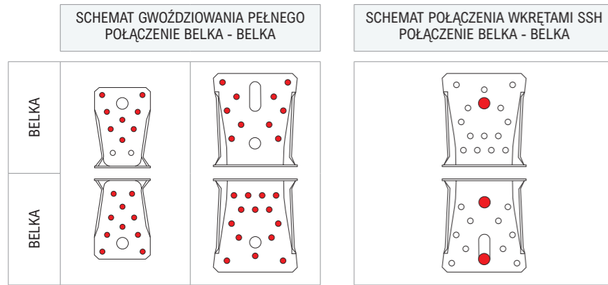
Połączenie krzyżowe dwóch elementów drewnianych za pomocą kątownika ABR100.
