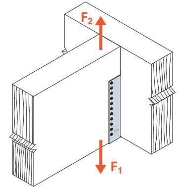
SCHEMAT OBCIĄŻENIA połączenie belka-belka
