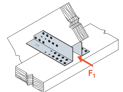
SCHEMAT OBCIĄŻENIA połączenie krokiew-murlata
