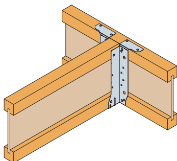
Połączenie belka dwuteowa do belki dwuteowej
