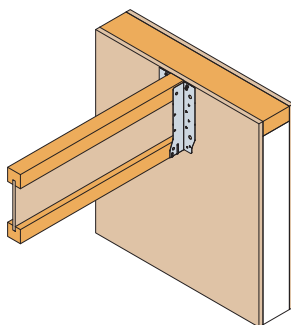
Połączenie belka dwuteowa do paneli SIP
