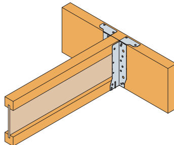
Połączenie belka dwuteowa do belki litej
